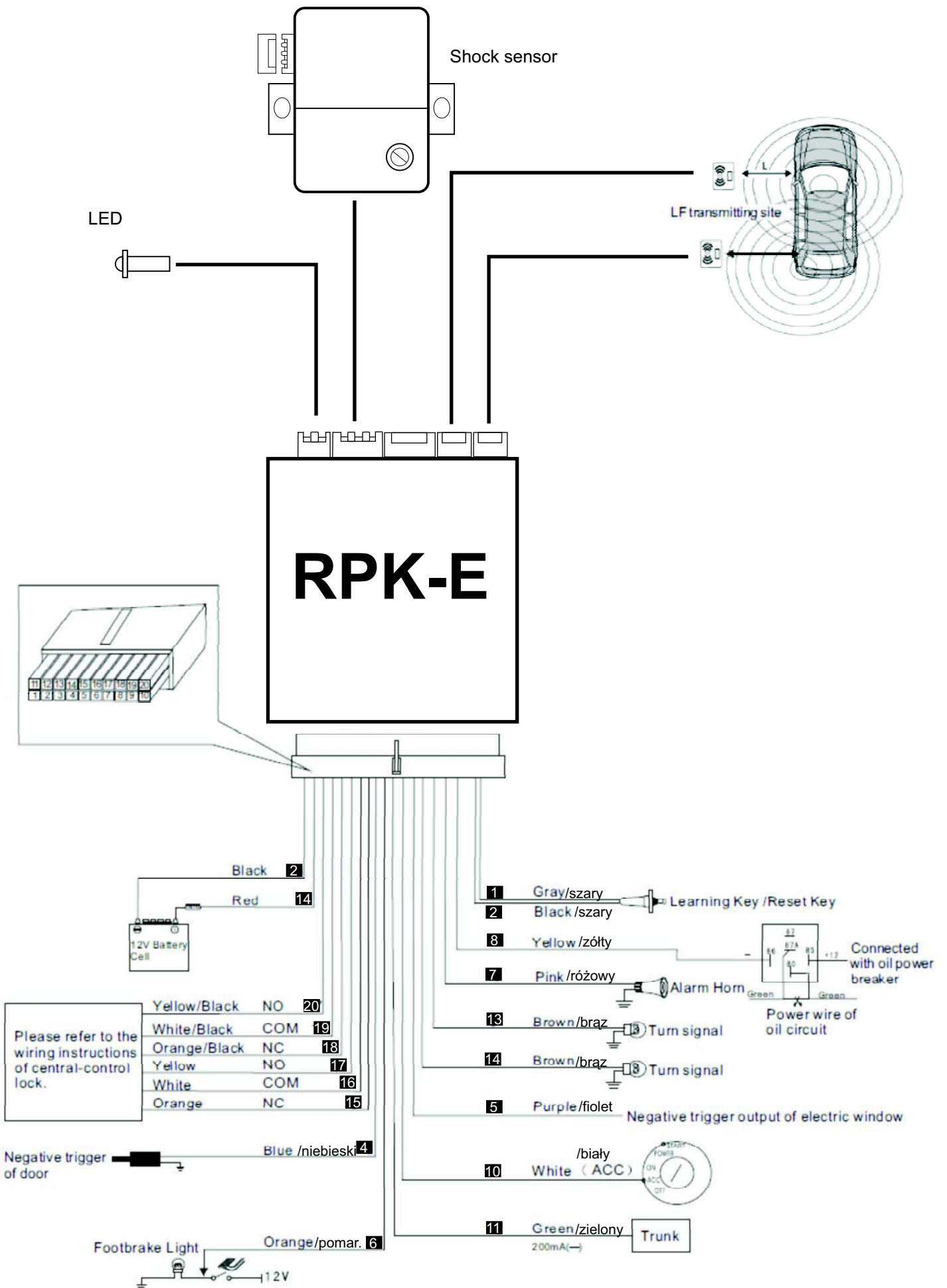
Schemat podłączenia alarmu R-PKE
